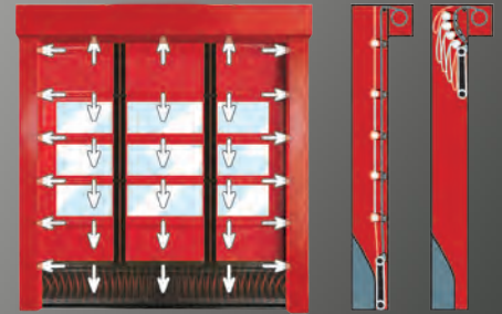
Распределение ветровой нагрузки
